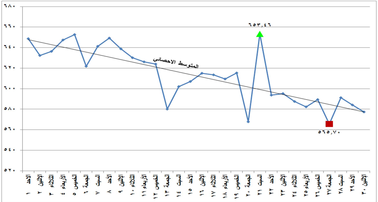
شكل (١٥) إجمالي الطاقة الكهربائية المنتجة من كل المصادر الأولية خلال شهر سبتمبر ٢٠١٩
