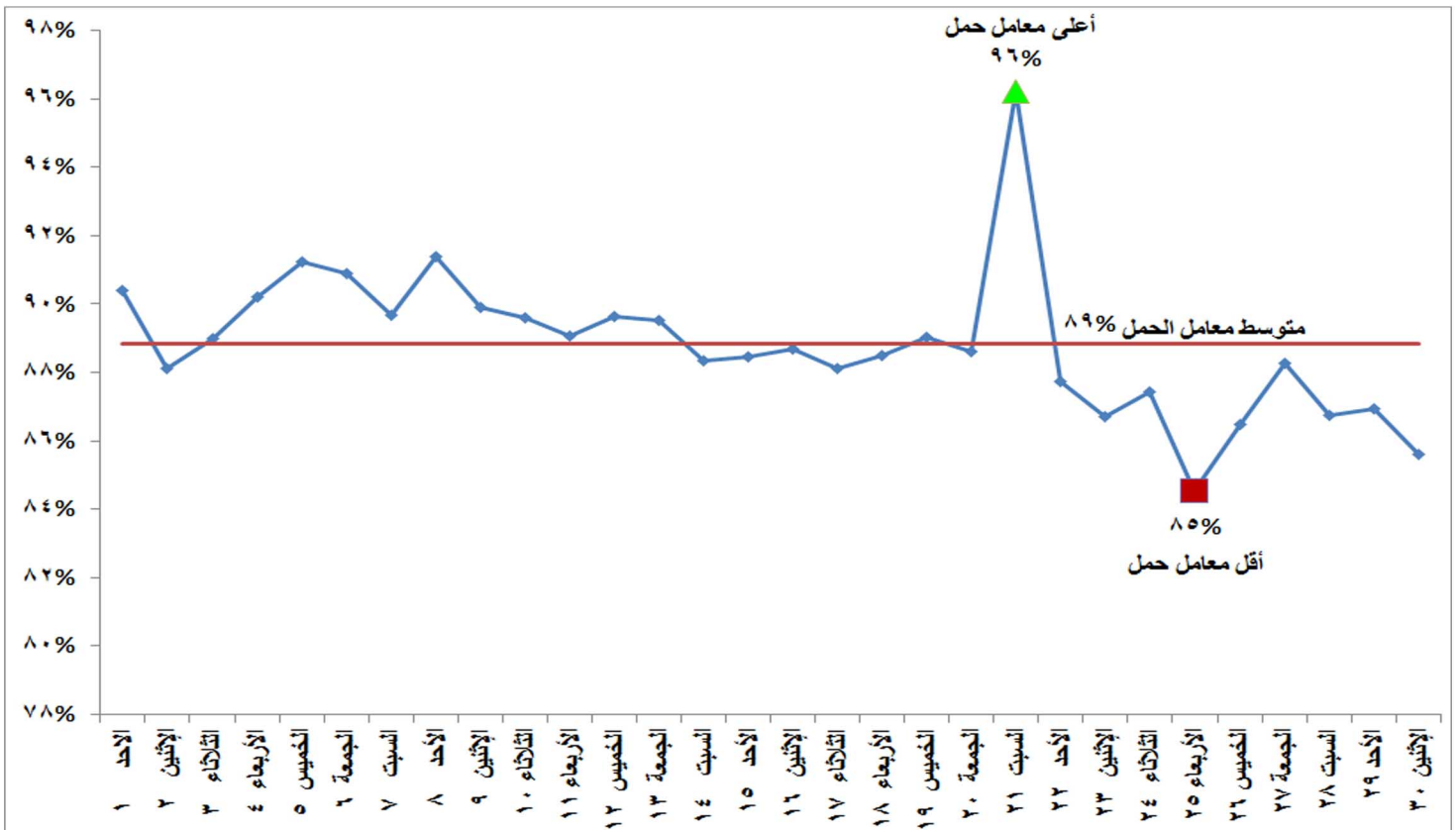
شكل (١٢) إجمالي معامل الحمل لوحدات الانتاج خلال شهر سبتمبر ٢٠١٩
