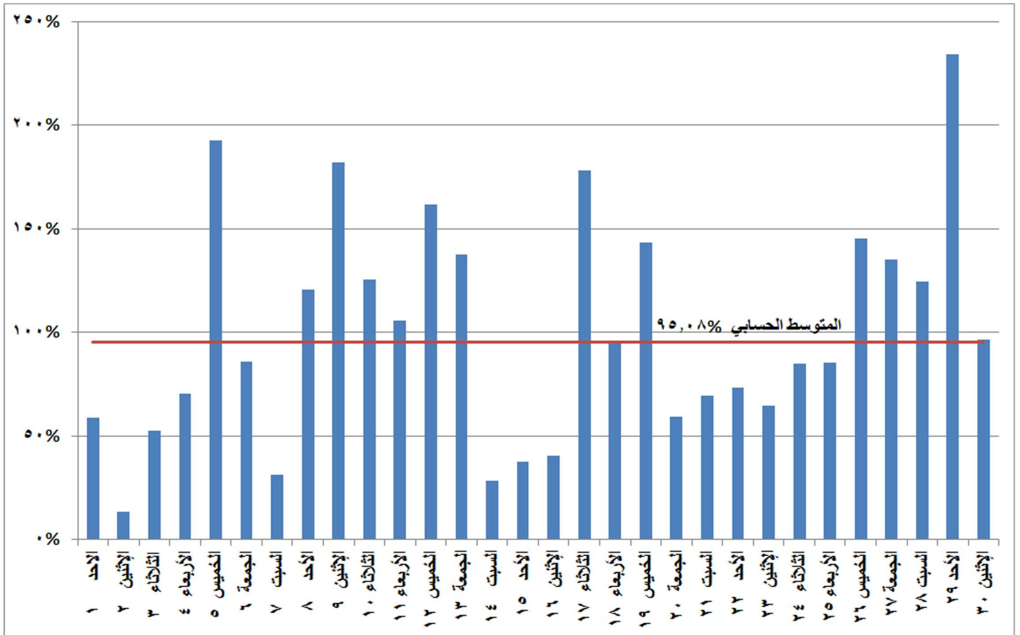
شكل (٢٦) نسب التغير في استخدام الرياح والشمس في إنتاج الطاقة الكهربائية خلال شهر سبتمبر ٢٠١٩ مقارنة بالشهر المماثل من العام السابق
