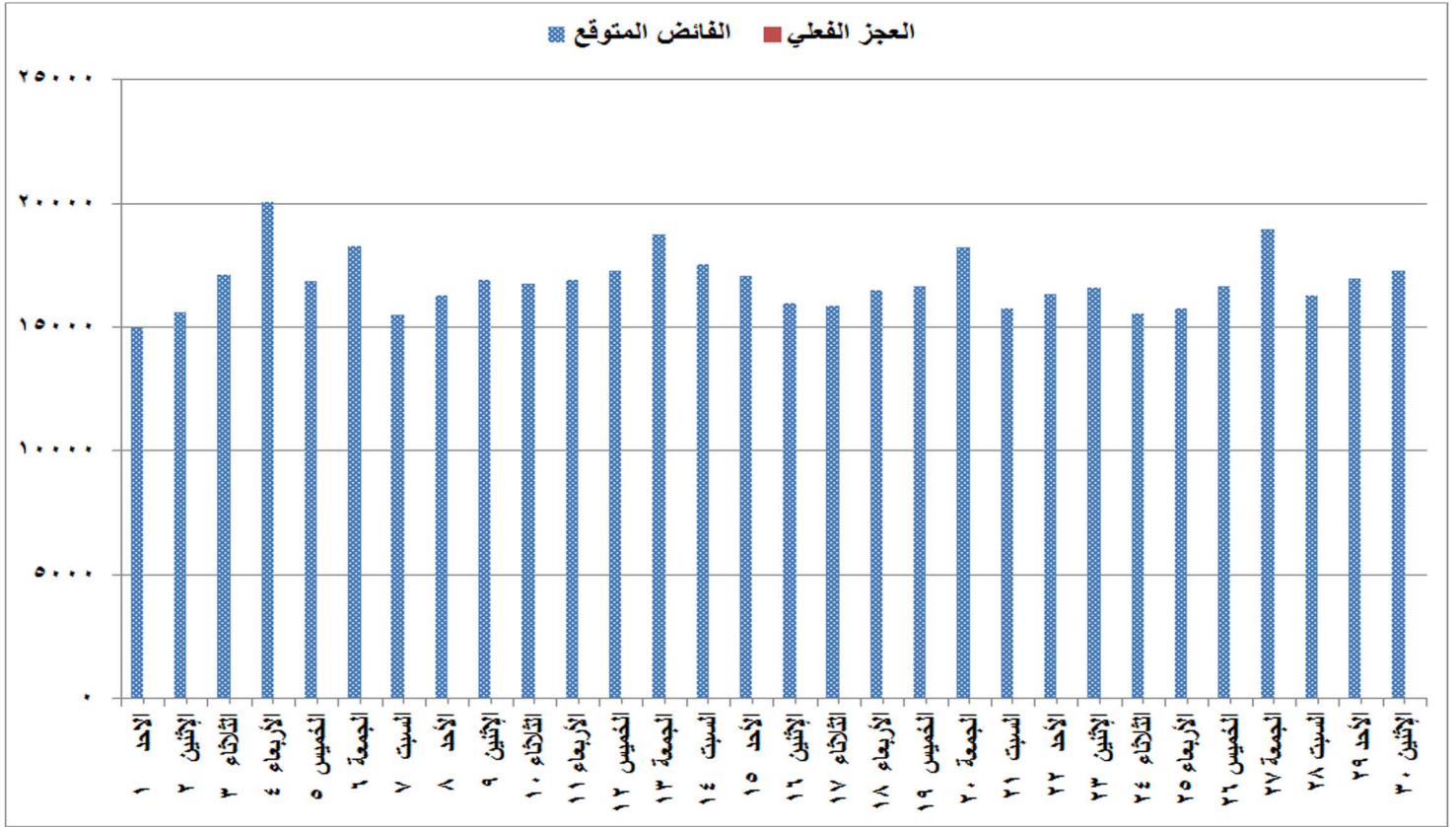
شكل (٧) الفائض والعجز المتوقع للقدرات خلال شهر سبتمبر ٢٠١٩
