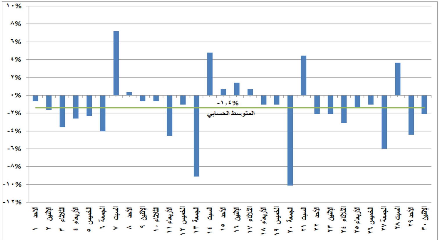
شكل (٩) النسب المئوية للتغير في الحمل الاقصى خلال شهر سبتمبر ٢٠١٩ مقارنة باليوم المماثل من العام الماضي
