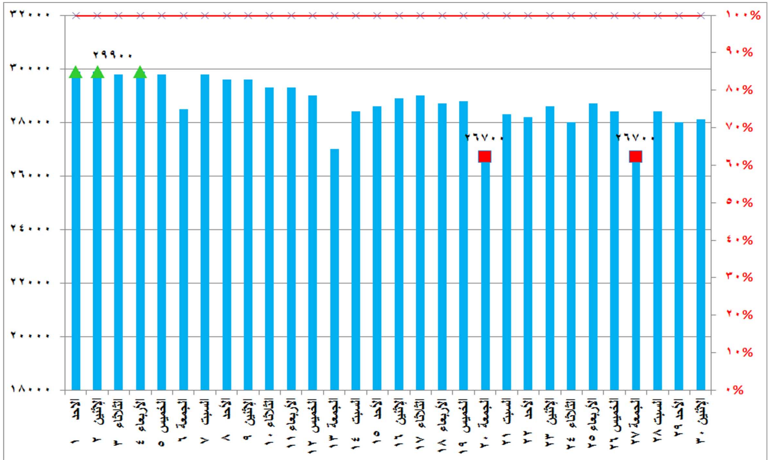
شكل (٥) قدرات الانتاج المتاحة ونسبتها للحمل الأقصى خلال شهر سبتمبر ٢٠١٩
