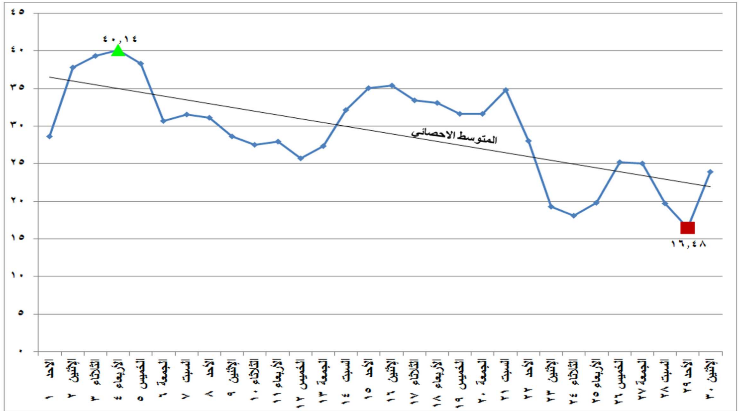
شكل (١٩) الطاقة الكهربائية المنتجة من المازوت خلال شهر سبتمبر ٢٠١٩
