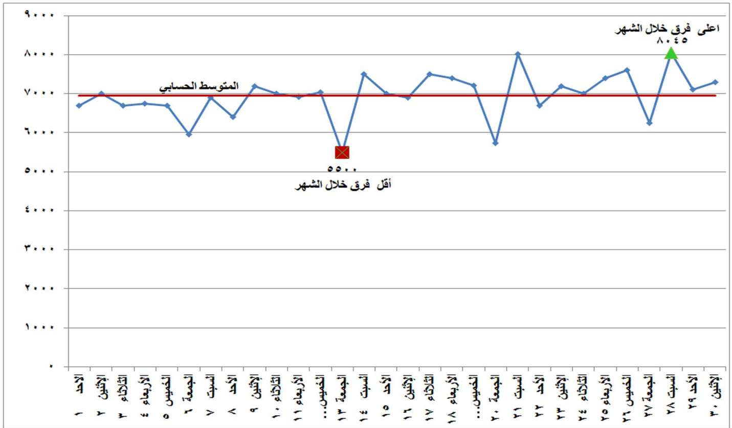
شكل (٣) الفرق بين أقصى وأدنى حمل خلال شهر سبتمبر ٢٠١٩
