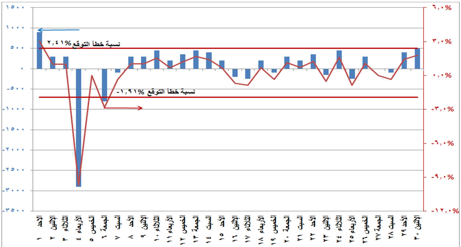
شكل (١٠) الفرق بين الحمل الأقصى المتوقع والمسجل فعليا ونسبة الفرق إلى الحمل المسجل فعليا خلال شهر سبتمبر ٢٠١٩
