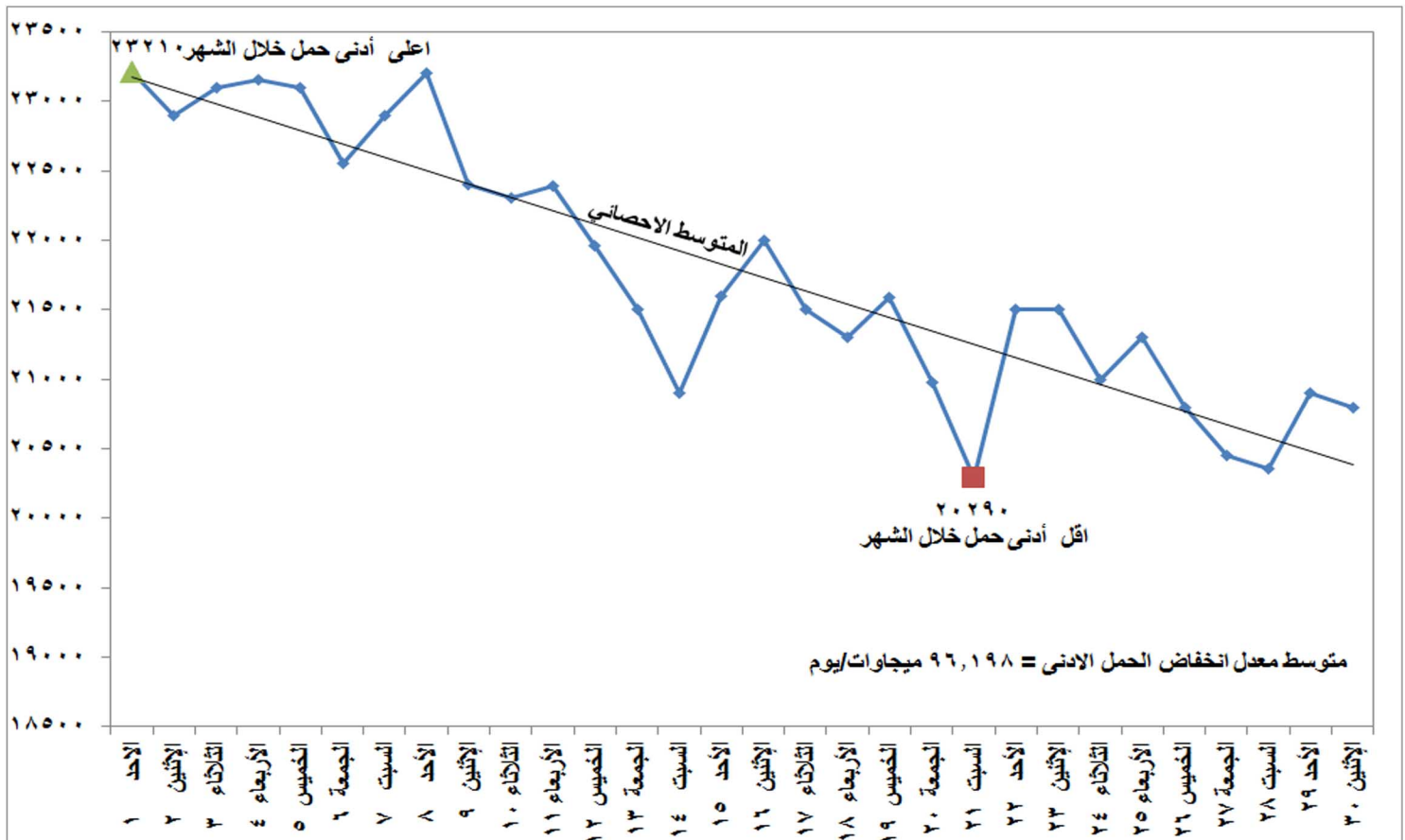
شكل (٢) تطور الحمل الادنى اليومي خلال شهر سبتمبر ٢٠١٩
