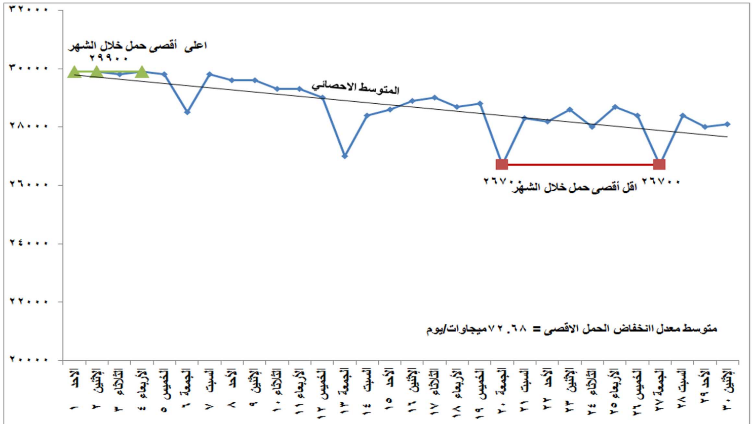
شكل (١) تطور الحمل الاقصى اليومي خلال شهر سبتمبر ٢٠١٩
