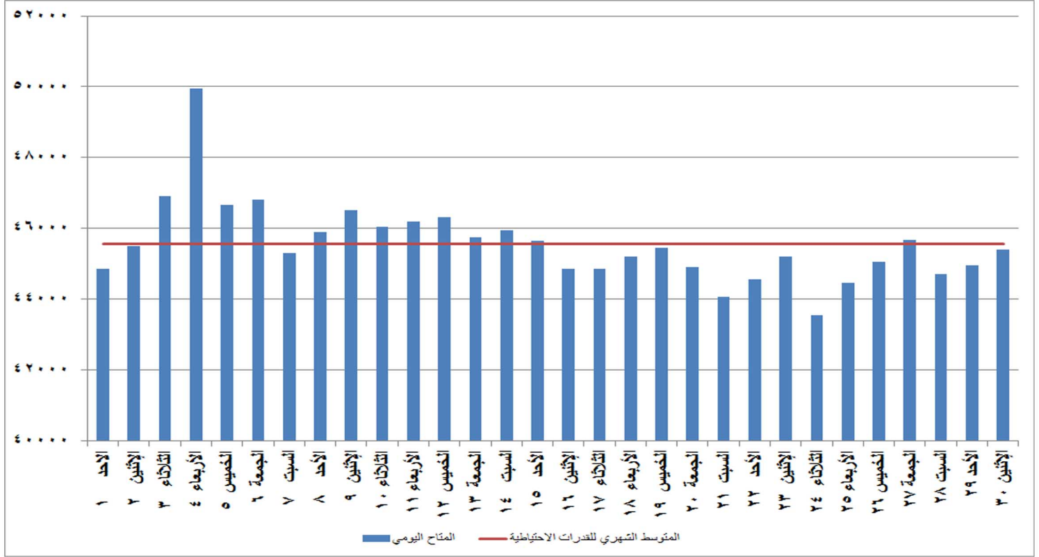
شكل (٢٧) القدرات المتاحة يوميا والمتوسط الشهري للقدرة الاحتياطية خلال شهر سبتمبر ٢٠١٩
